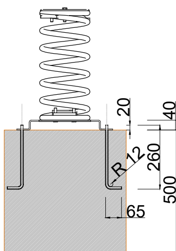
Alçado , Esquema de Fixação
