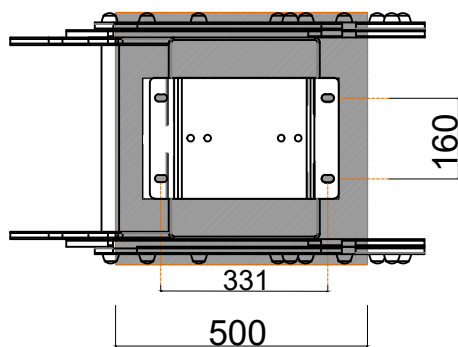
PLANTA, Esquema de Fixação
