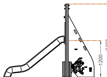
ALÇADO LATERAL SIDE VIEW
