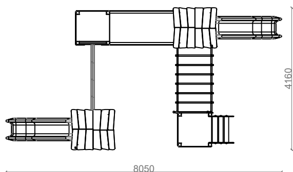
PLANTA PLAN
