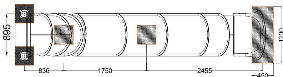
PLANTA . ESQUEMA DE FIXAÇÃO PLAN . INSTALLATION PLAN
