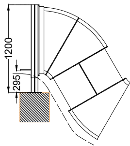
ALÇADO . ESQUEMA DE FIXAÇÃO SIDE VIEW . INSTALLATION PLAN
