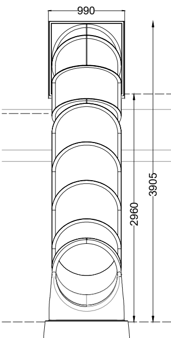
ALÇADO FRONTAL FRONT VIEW
