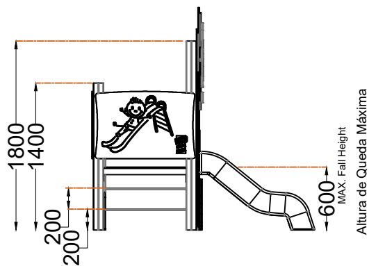
ALÇADO LATERAL SIDE VIEW
