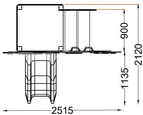
PLANTA PLAN
