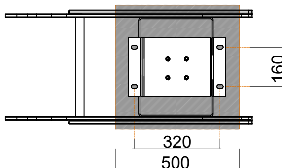
PLANTA, Esquema de Fixação
