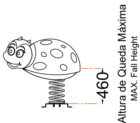
ALÇADO LATERAL SIDE VIEW
