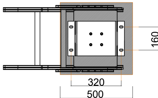
PLANTA, Esquema de Fixação
