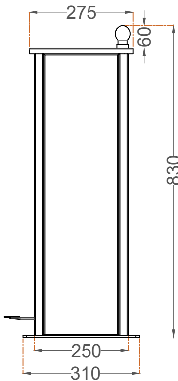
ALÇADO LATERAL SIDE VIEW
