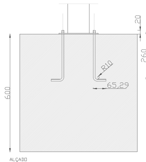
ALÇADO
