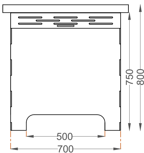
ALÇADO FRONTAL FRONT VIEW
