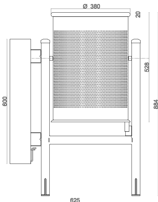
ALÇADO FRONTAL
