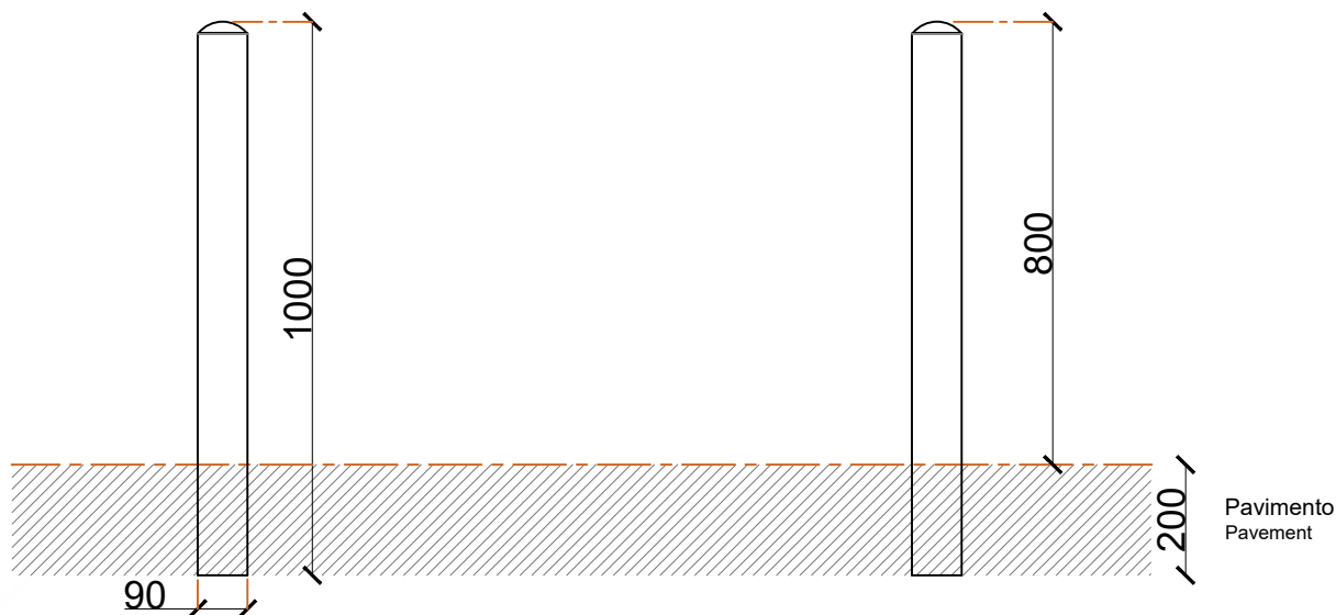
ALÇADO LATERAL SIDE VIEW
