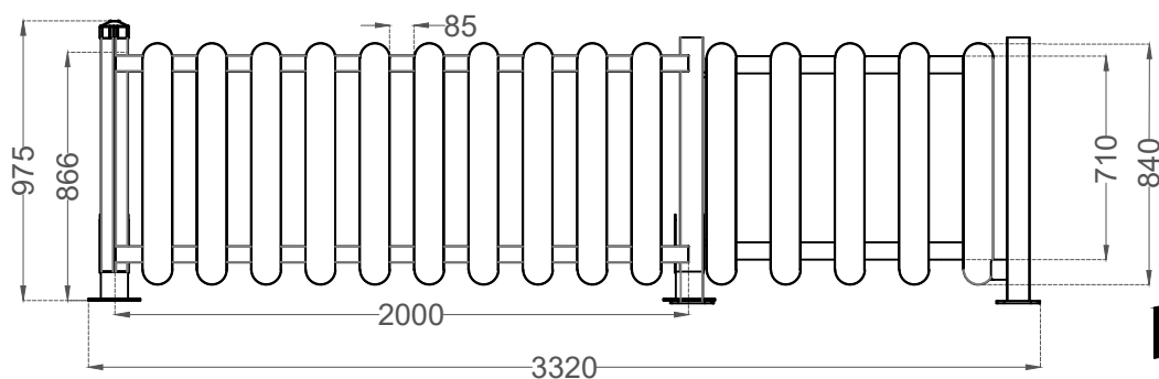
ALÇADO FRONTAL FRONT VIEW
