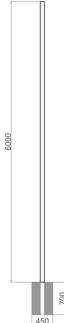
PLANTA . ESQUEMA DE MACIÇOS
