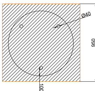
PLANTA . ESQUEMA DE MACIÇOS
