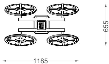
PLANTA PLAN
