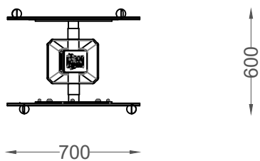
PLANTA PLAN
