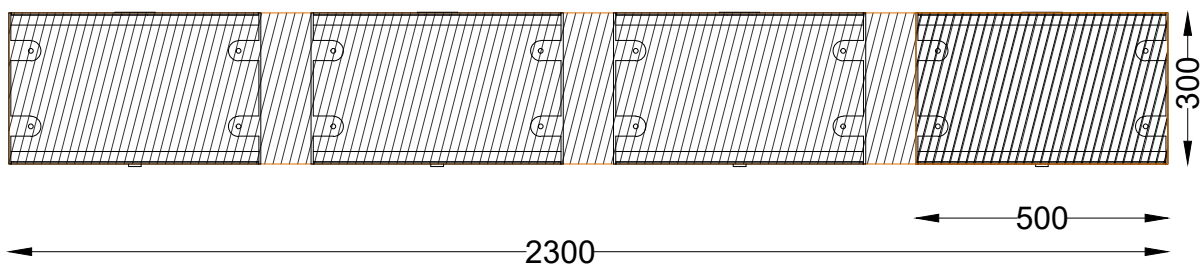
PLANTA . ESQUEMA DE FIXAÇÃO PLAN . INSTALLATION PLAN
