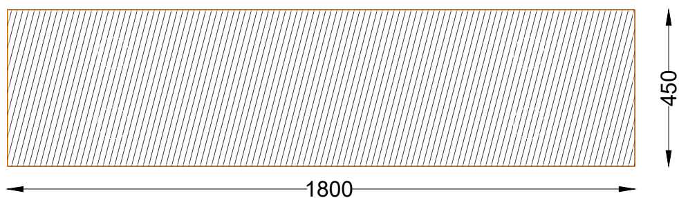
PLANTA . ESQUEMA DE FIXAÇÃO PLAN . INSTALLATION PLAN
