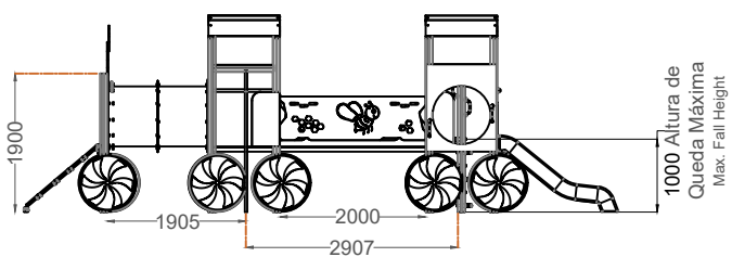
ALÇADO LATERAL SIDE VIEW
