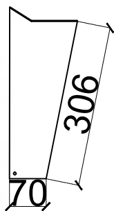
ALÇADO LATERAL SIDE VIEW
