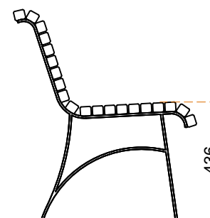
ALÇADO LATERAL
