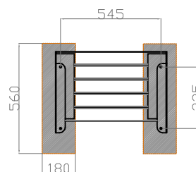
PLANTA - ESQUEMA DE MACIÇOS
