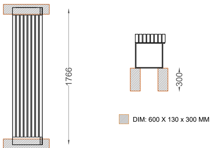
PLANTA . ESQUEMA DE FIXAÇÃO PLAN . INSTALLATION PLAN
