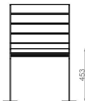
ALÇADO FRONTAL
