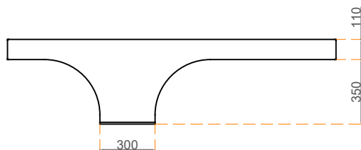
ALÇADO FRONTAL
