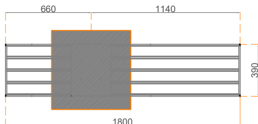
PLANTA . ESQUEMA MACIÇO
