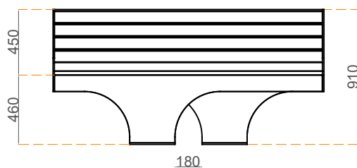
ALÇADO FRONTAL
