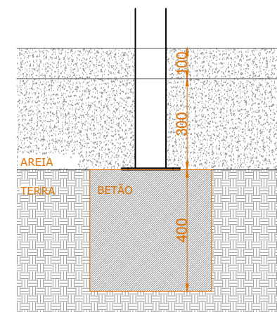
ESQUEMA DE FIXAÇÃO (PISO DE AREIA)
