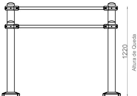
ALÇADO - INDICAÇÃO DA ALTURA DE QUEDA
