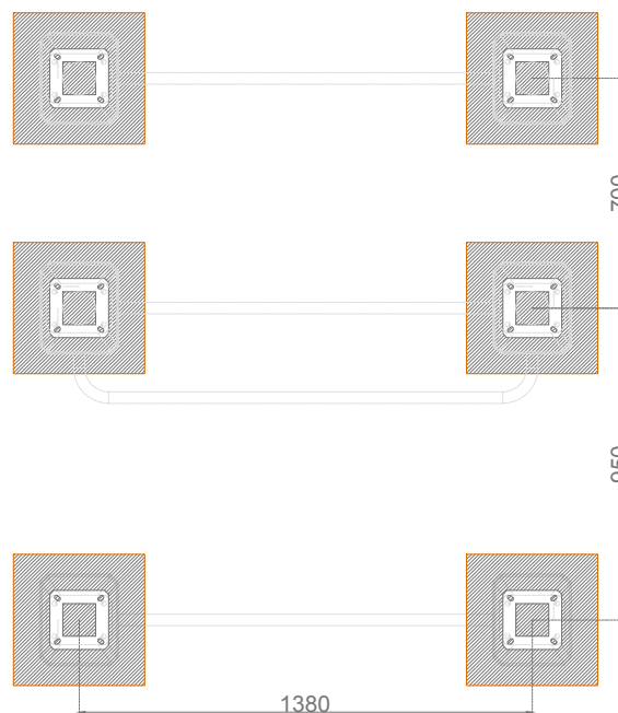
PLANTA . ESQUEMA DE MACIÇOS
