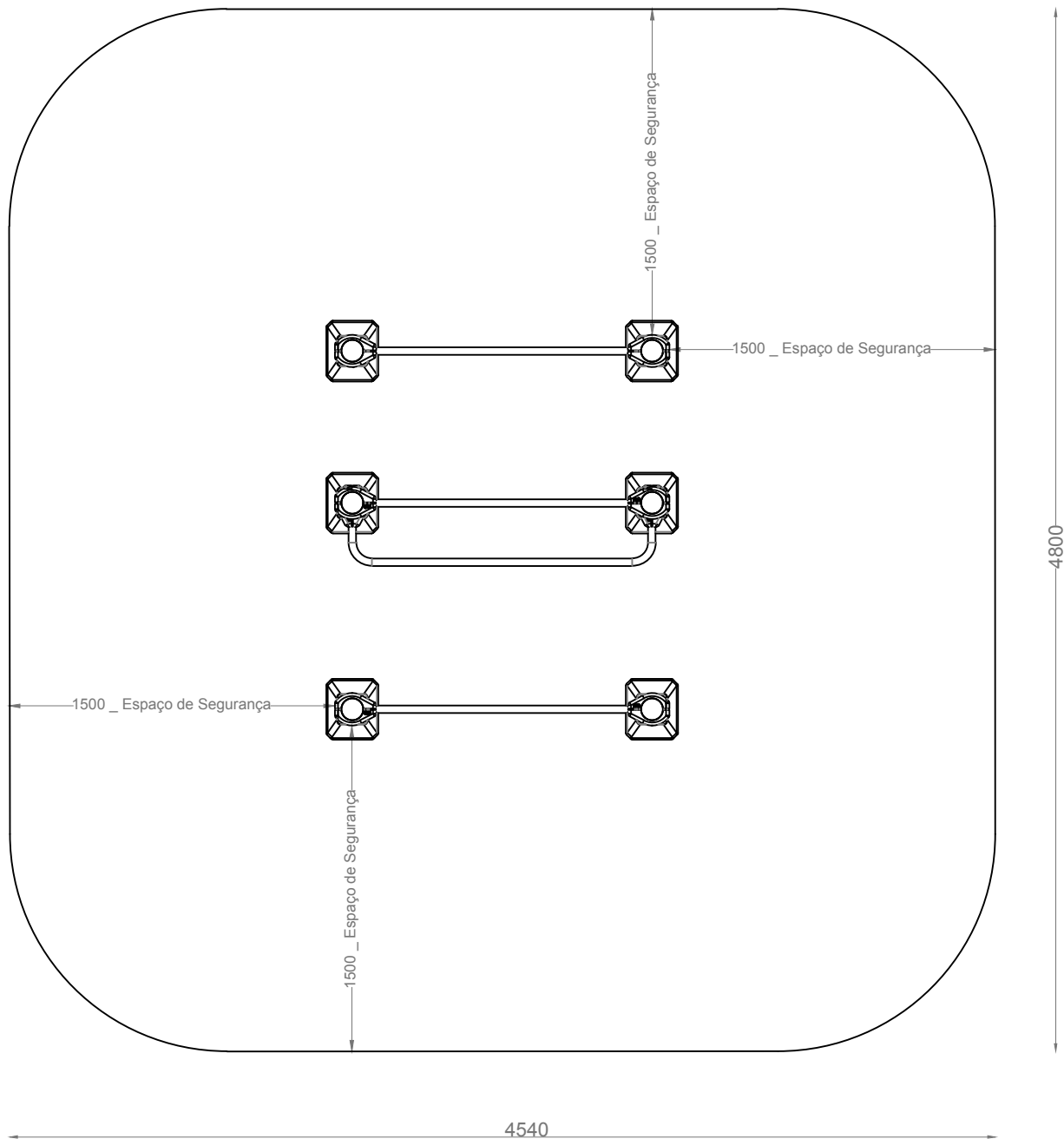
PLANTA - ENQUADRAMENTO DO EQUIPAMENTO NO ESPAÇO DE SEGURANÇA NECESSÁRIO
