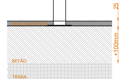
ESQUEMA DE FIXAÇÃO (PISO SINTÉTICO)
