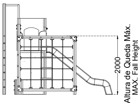
ALÇADO LATERAL SIDE VIEW
