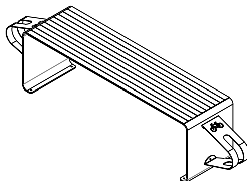
VISTA ISOMÉTRICA
