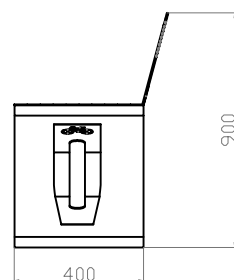
ALÇADO LATERAL
