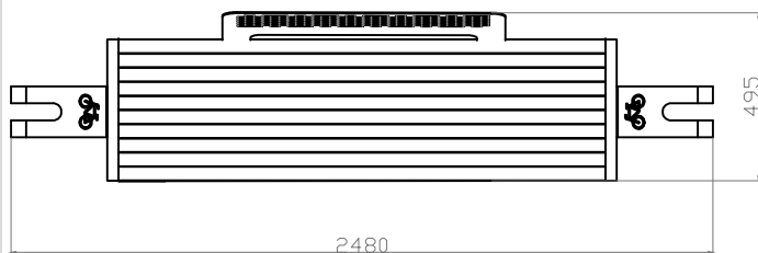
PLANTA
