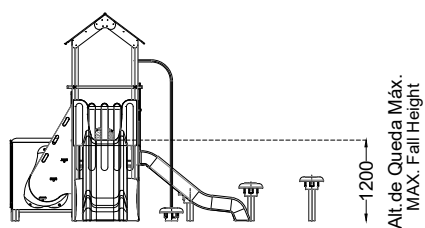
ALÇADO FRONTAL FRONT VIEW
