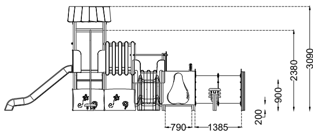
ALÇADO LATERAL SIDE VIEW
