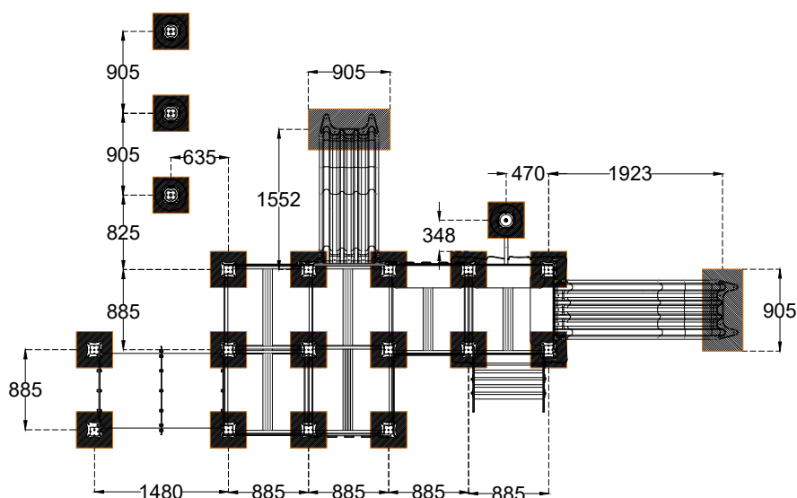
PLANTA . ESQUEMA DE FIXAÇÃO PLAN . INSTALLATION PLAN
