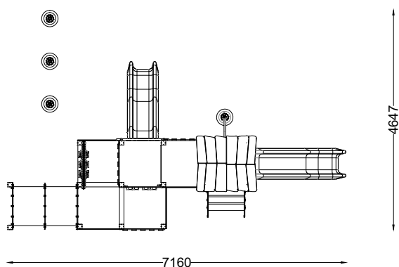
PLANTA PLAN
