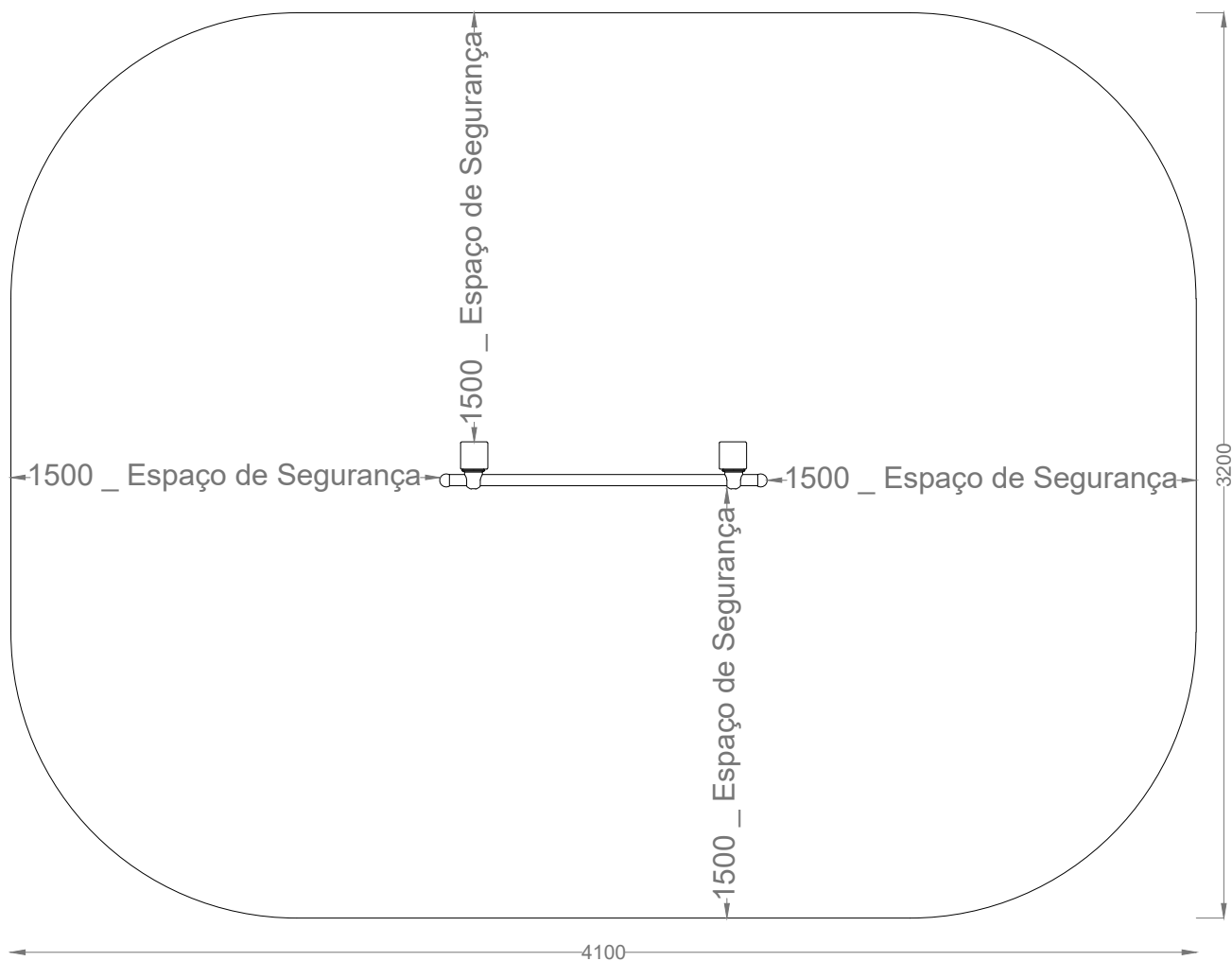
PLANTA - ENQUADRAMENTO DO EQUIPAMENTO NO ESPAÇO DE SEGURANÇA NECESSÁRIO
