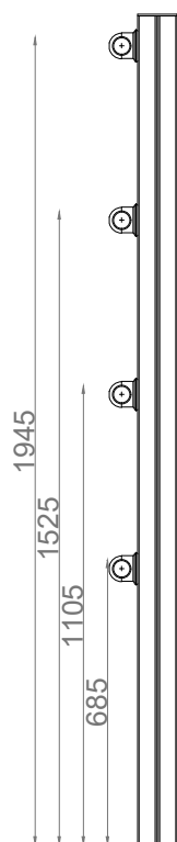
ALÇADO LATERAL
