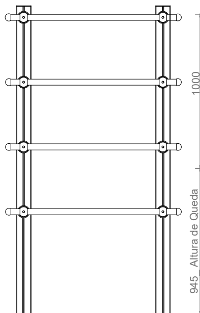
ALÇADO - INDICAÇÃO DA ALTURA DE QUEDA
