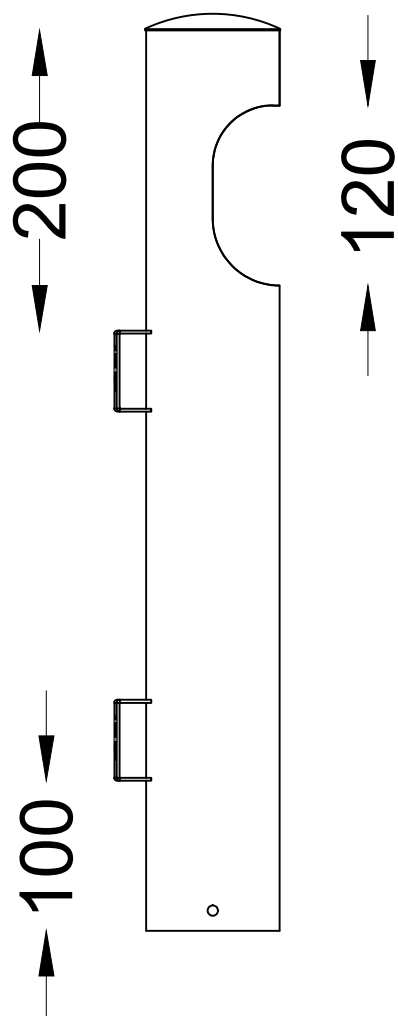
ALÇADO LATERAL SIDE VIEW
