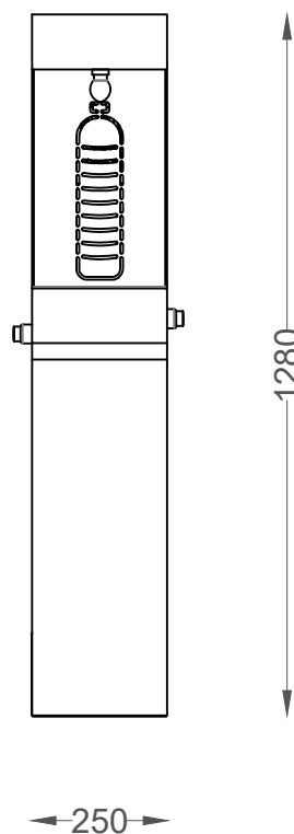
ALÇADO FRONTAL FRONT VIEW
