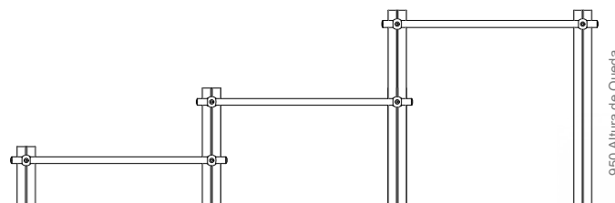
ALÇADO - INDICAÇÃO DA ALTURA DE QUEDA
