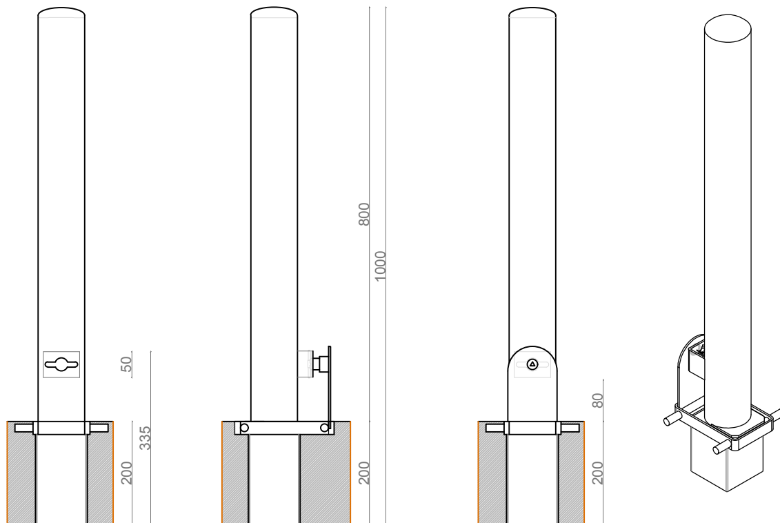
ALÇADO FRONTAL (sem peça de fixação)
