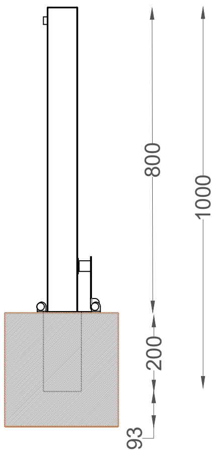
ALÇADO LATERAL SIDE VIEW
