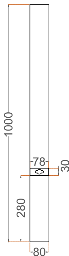
POSTE POST
