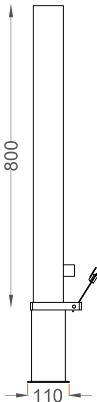
ALÇADO LATERAL SIDE VIEW
