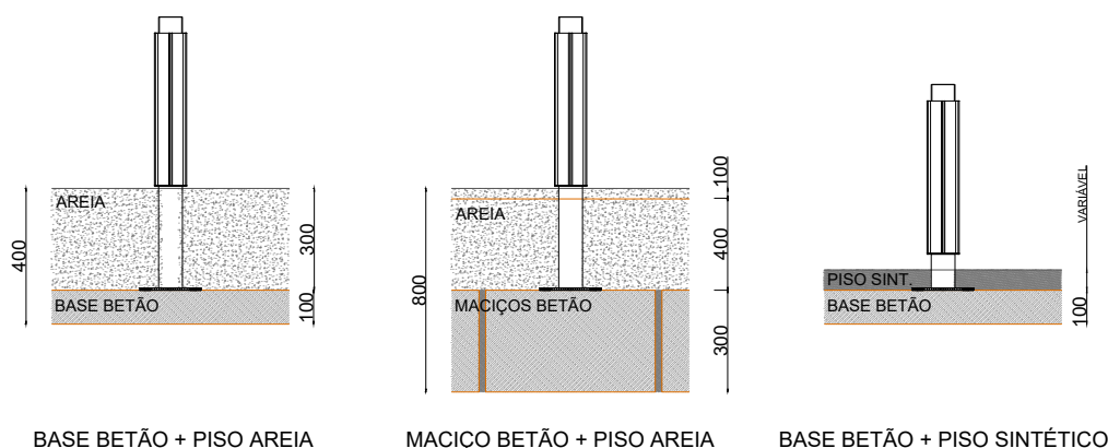
PLANTA . ESQUEMA DE FIXAÇÃO PLAN . INSTALLATION PLAN
