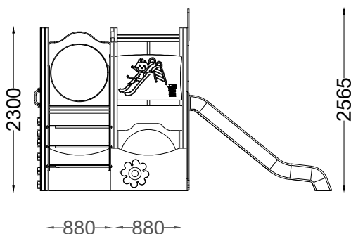
ALÇADO FRONTAL FRONT VIEW
