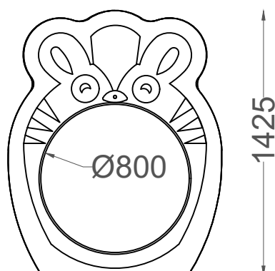
ALÇADO FRONTAL FRONT VIEW
