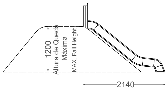
ALÇADO LATERAL SIDE VIEW
