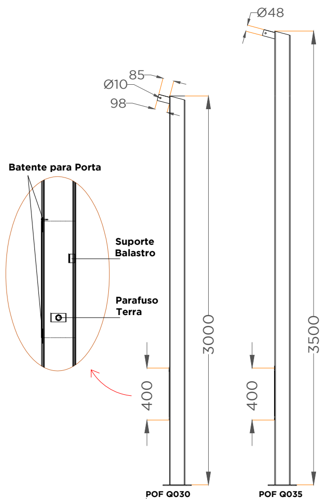
ALÇADO LATERAL SIDE VIEW
