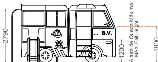
ALÇADO LATERAL SIDE VIEW
