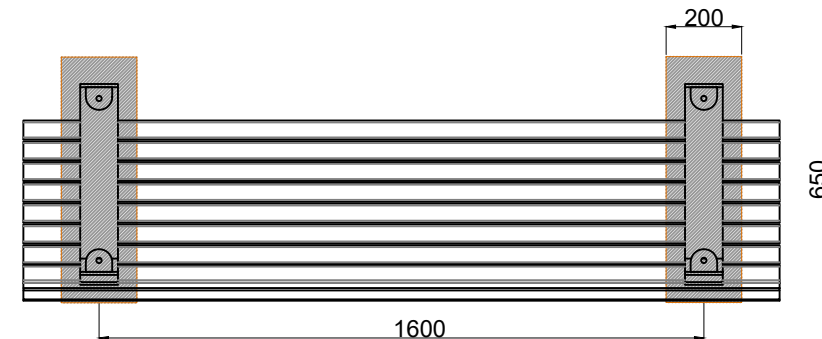
PLANTA . ESQUEMA DE MACIÇOS
