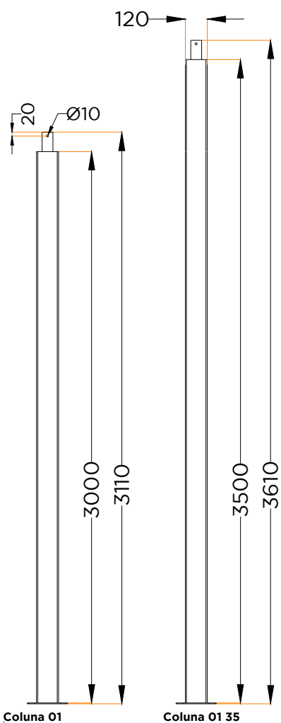
ALÇADO LATERAL SIDE VIEW
