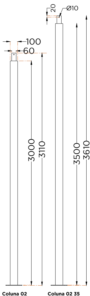
ALÇADO LATERAL SIDE VIEW
