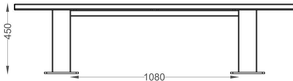
ALÇADO FRONTAL FRONT VIEW
