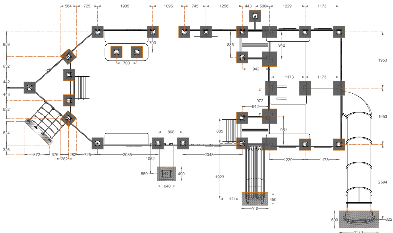
PLANTA . ESQUEMA DE FIXAÇÃO PLAN . INSTALLATION PLAN
