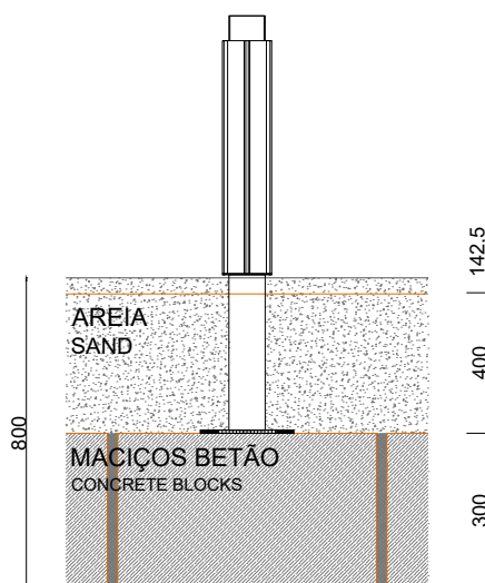
MACIÇO BETÃO + PISO AREIA CONCRETE BLOCK + SAND LAYER
