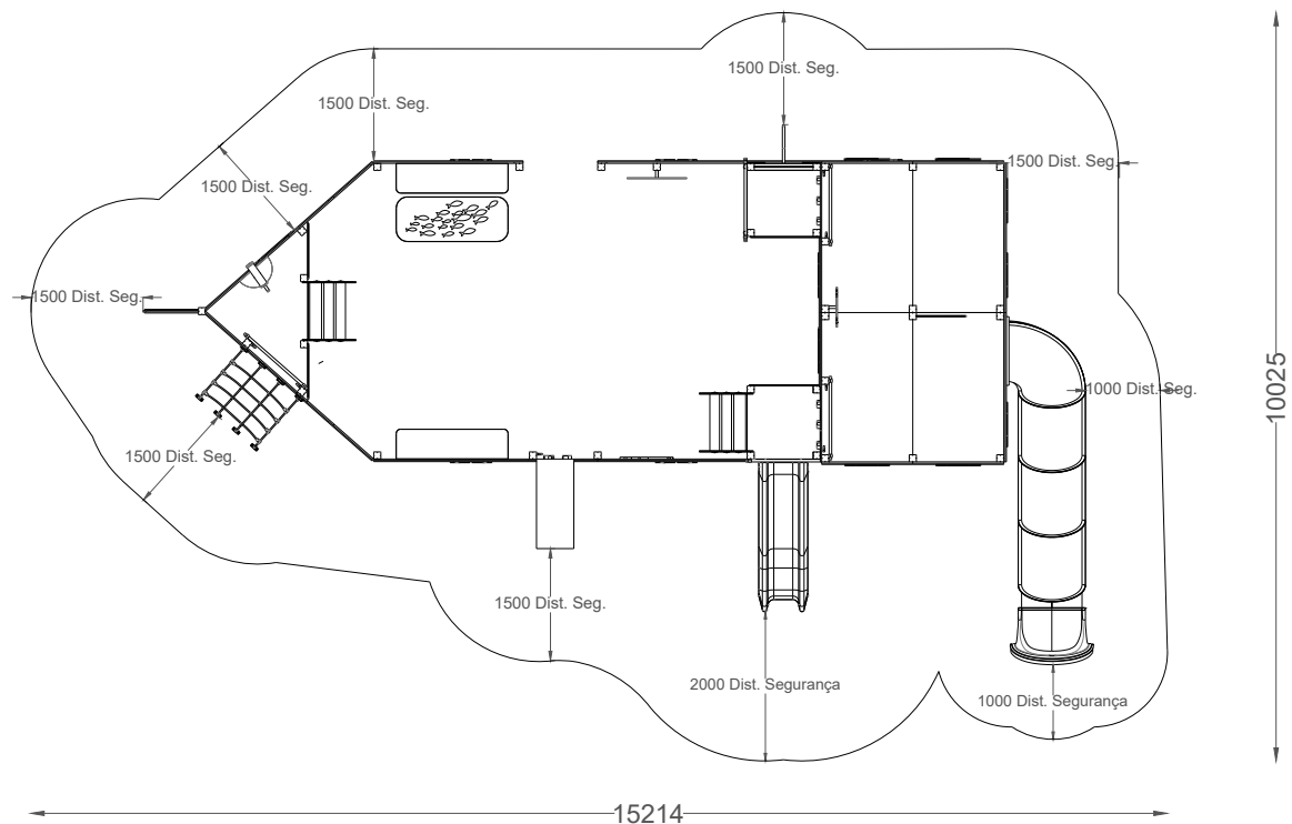
PLANTA - ESPAÇO DE SEGURANÇA NECESSÁRIO PLAN - SAFETY SPACE REQUIRED
