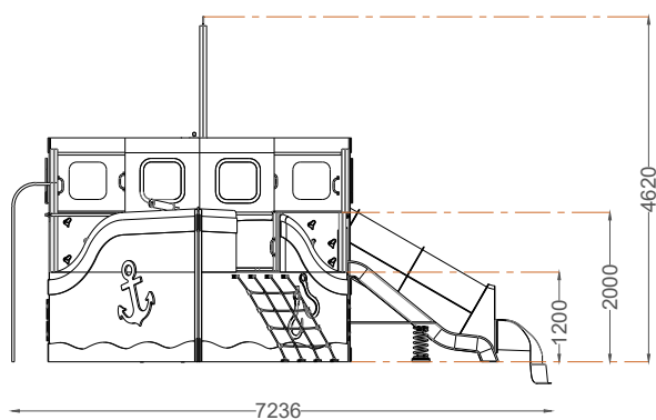
ALÇADO FRONTAL FRONT VIEW
