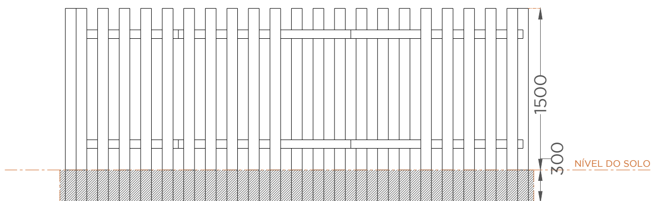
ALÇADO FRONTAL . ESQUEMA DE FIXAÇÃO FRONTAL VIEW . INSTALLATION PLAN
