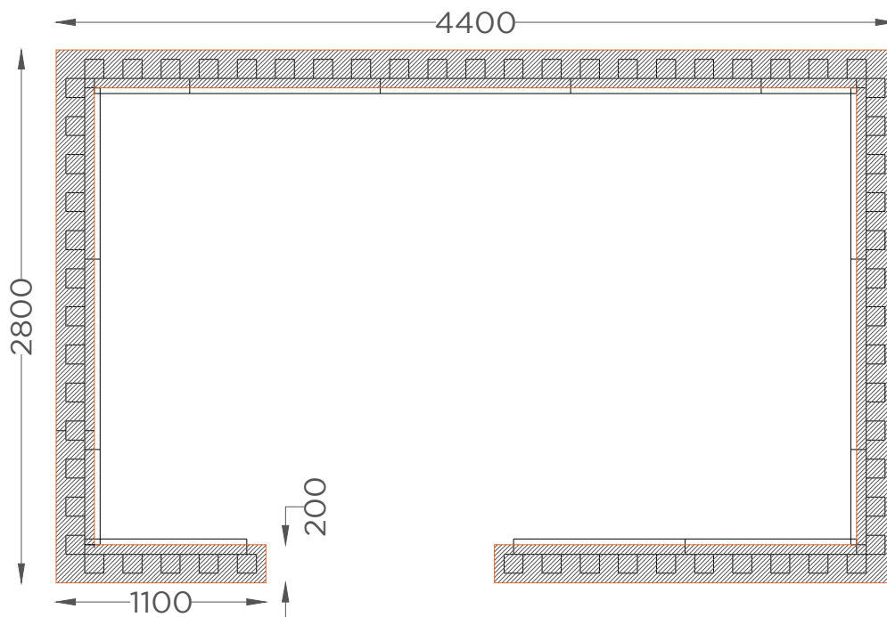
PLANTA . ESQUEMA DE FIXAÇÃO PLAN . INSTALLATION PLAN
