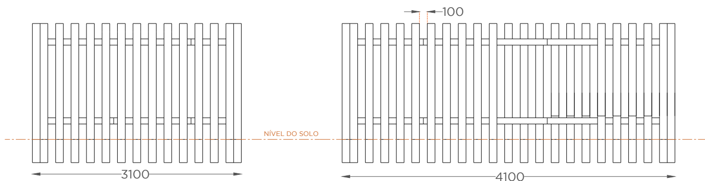
ALÇADO LATERAL SIDE VIEW
