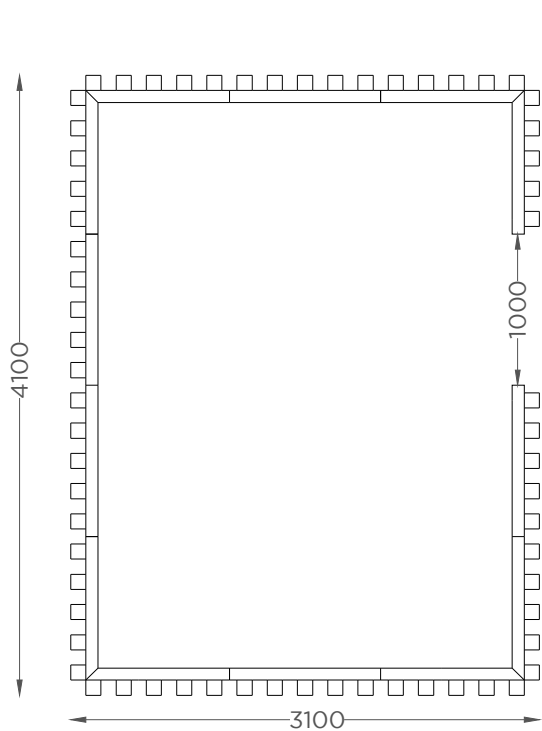
PLANTA PLAN
